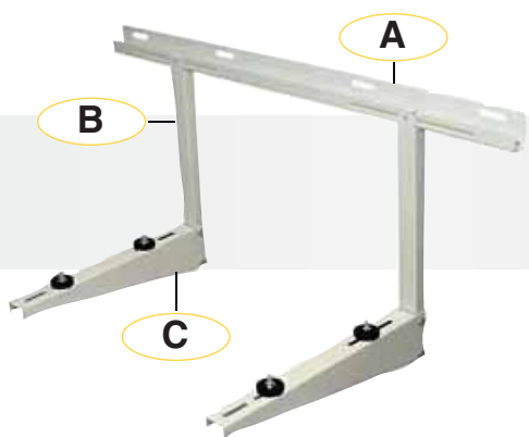
Veggfeste for utedel A= 800mm B=450mm C=450mm Kapasitet: 150 kg, vibrasjonsdempere følger med.
